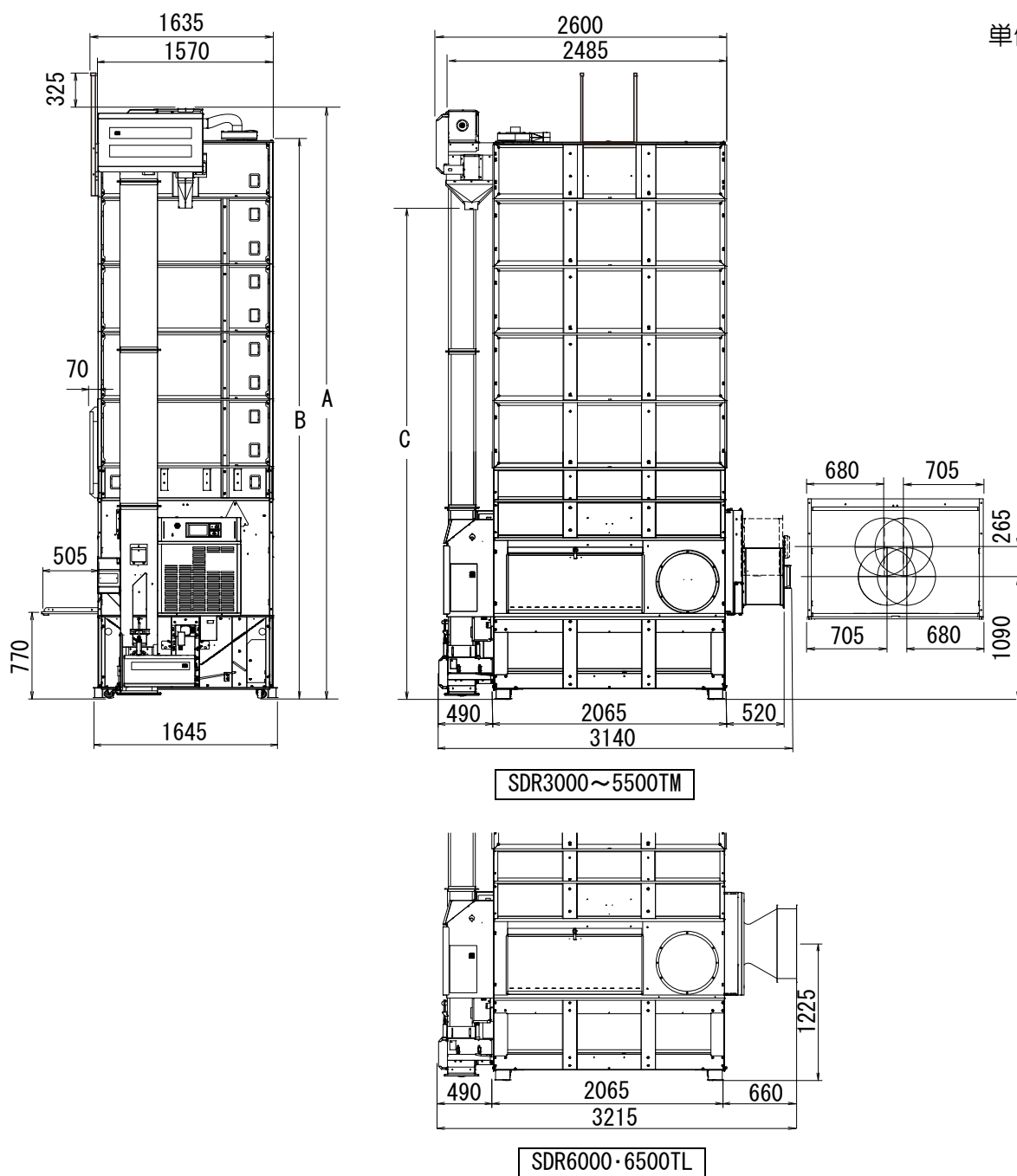
図 5 機体寸法
