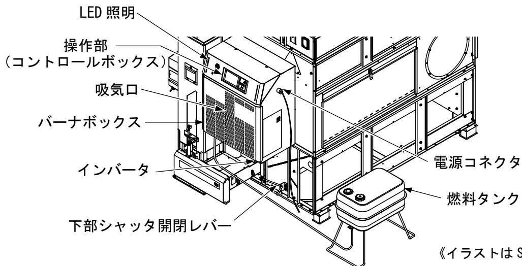
図 3 機械全体図 (1)
